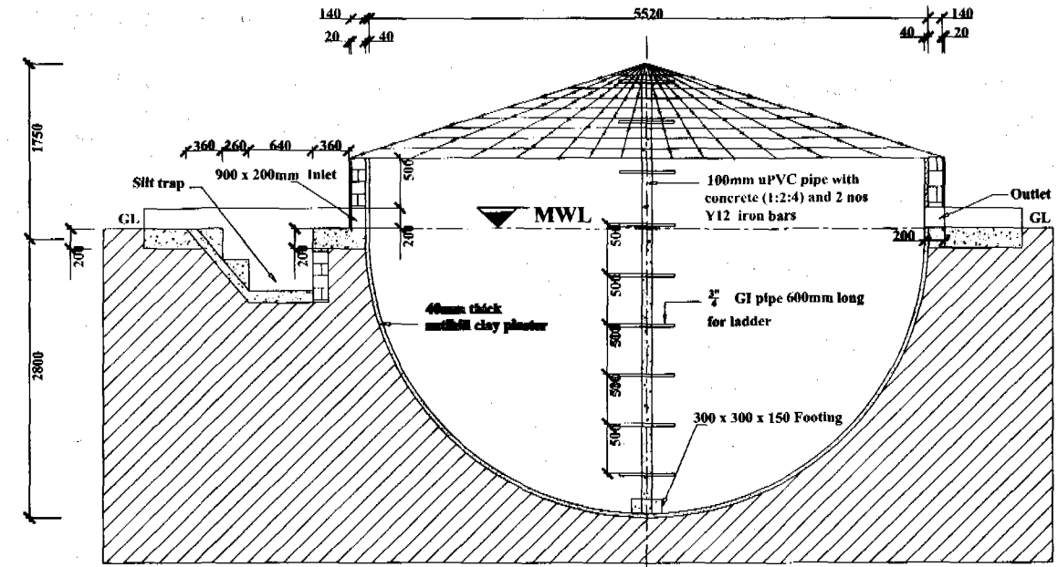
SECTION A-A (mm)
