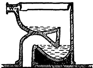
Fig. VI.16. Wash out closet.
