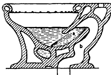
Fig. VI.19. Siphon jet closet.
