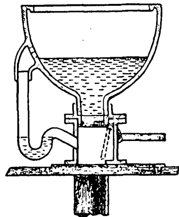
Fig. VI.12. Valve closet.
