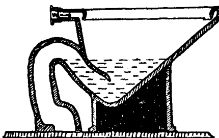
Fig. VI.18. Siphon closet.
