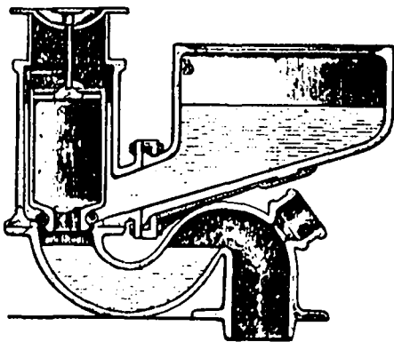
Fig. VI.13. Plunger closet.
