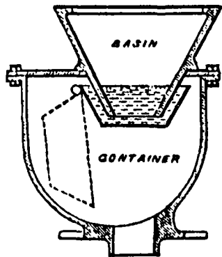
Fig. VI.11. Pan closet.
