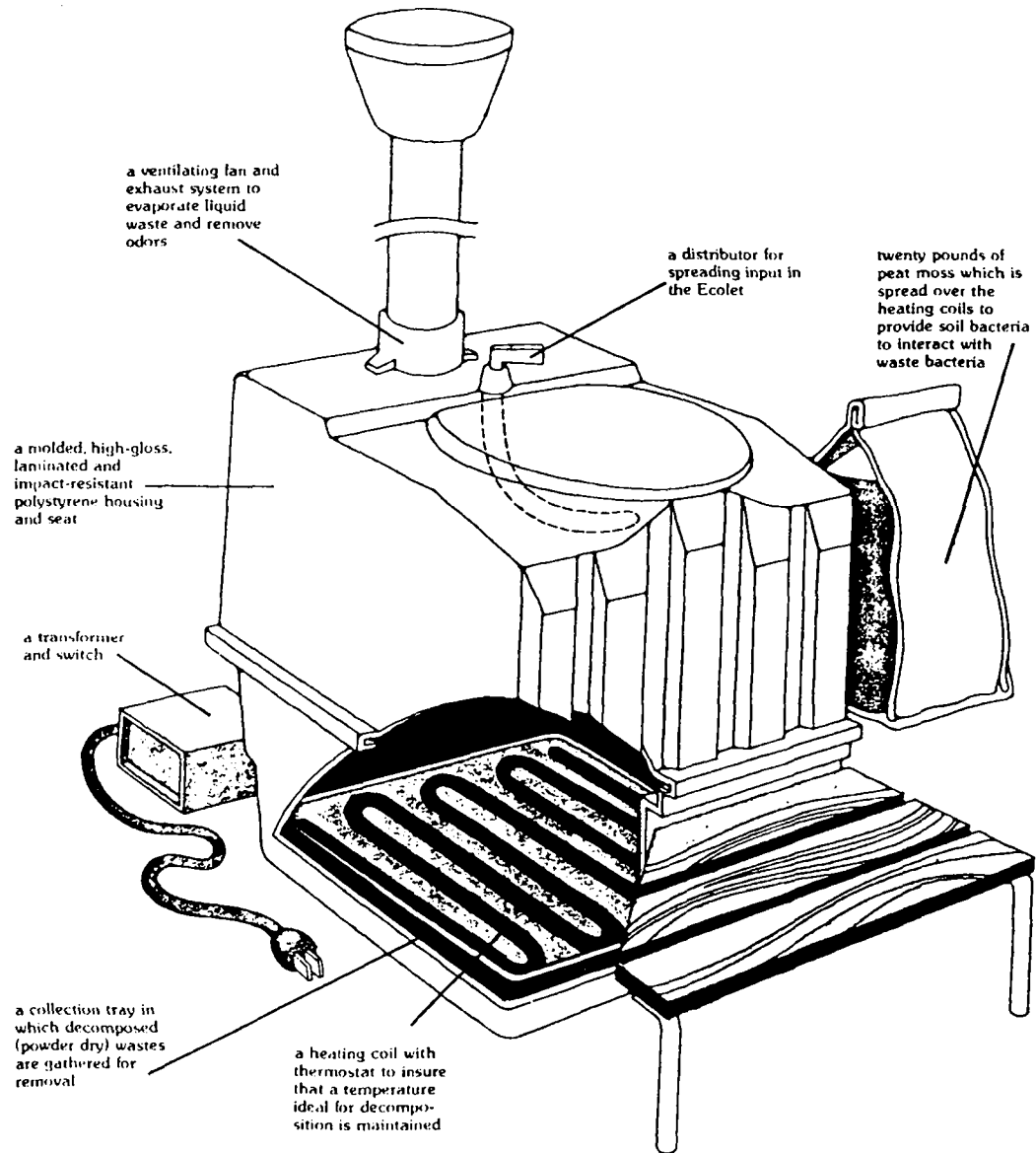
Fig. IX.12. Ecolet.
