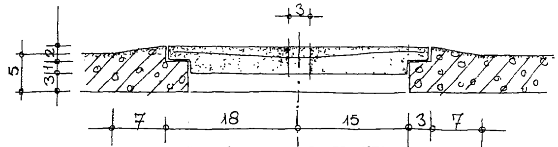
CORTE DEL AGUJERO CENTRAL EN LA PLANCHA, LA TAPADERA ESTÁ PUESTO EN EL LUGAR DE LA TAZA.
