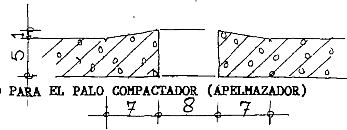
CORTE DEL AGUJERO CENTRAL EN LA PLANCHA, LA TAPADERA ESTÁ PUESTO EN EL LUGAR DE LA TAZA.
