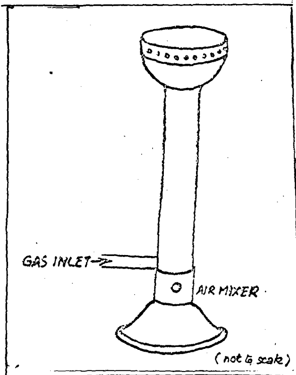
Fig. 44: Fischer's Burner
