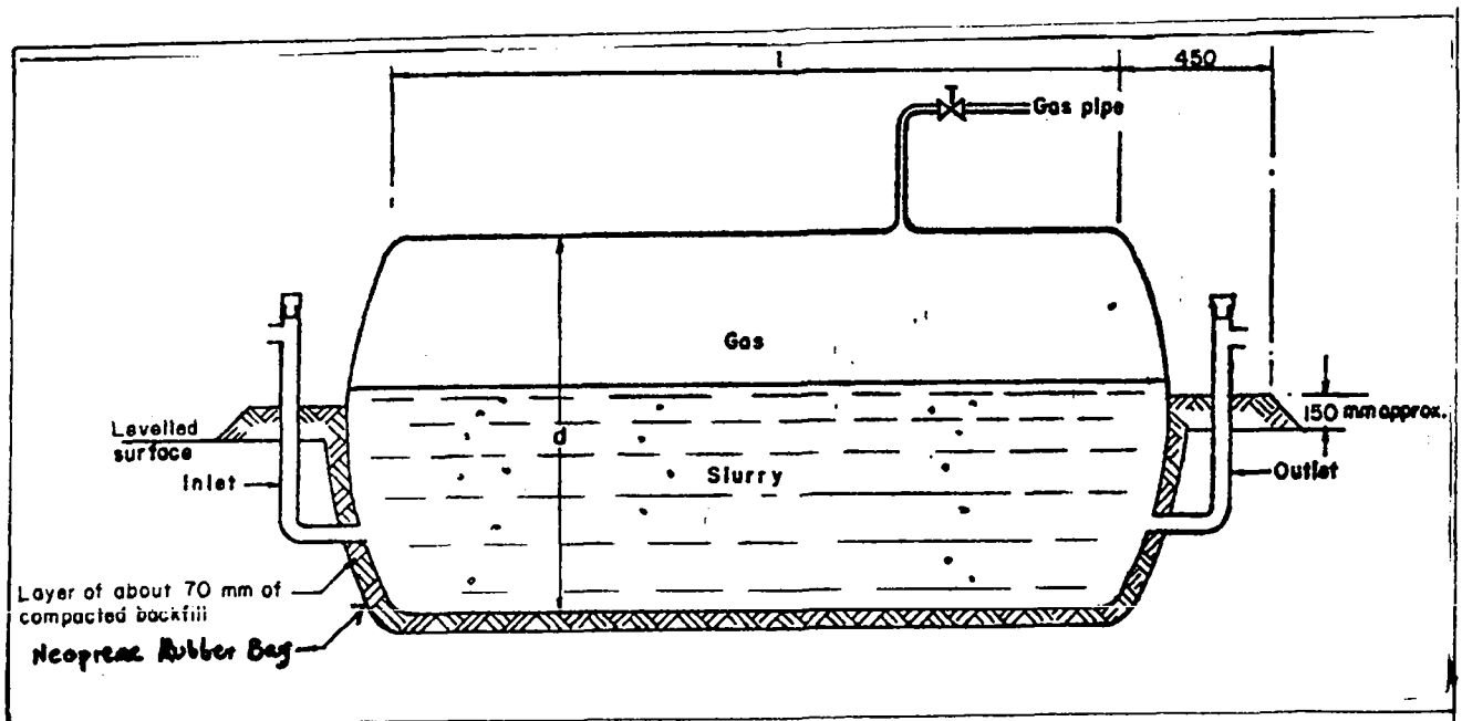
Fig. 29. Biogas Bag Digester
