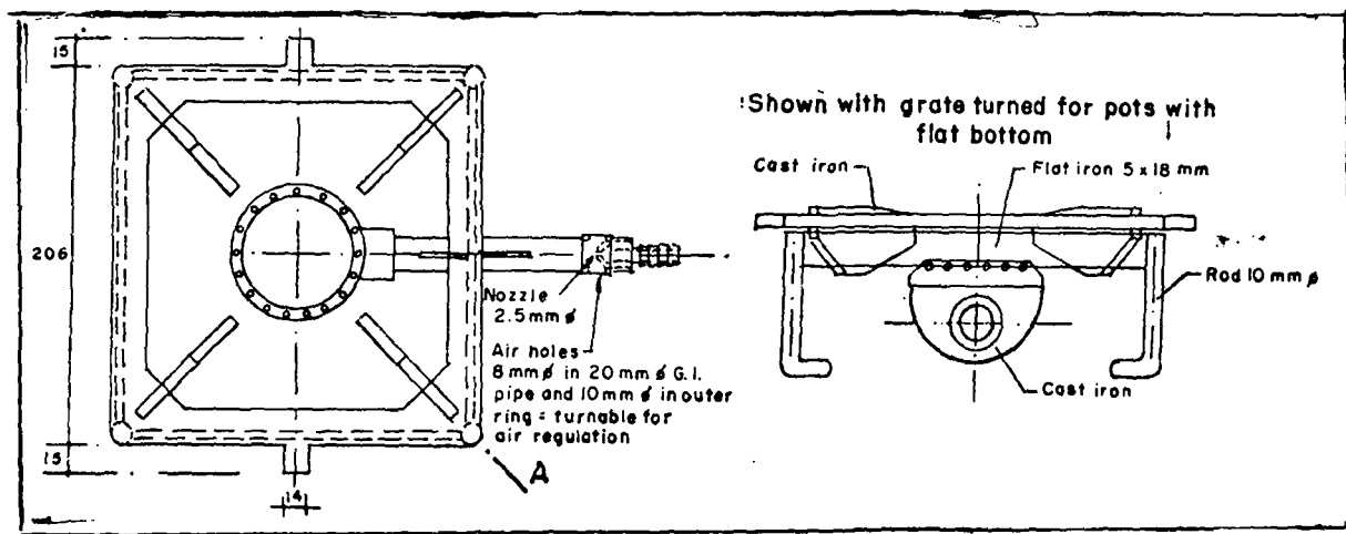
Fig. 53: Nepali Chulo
