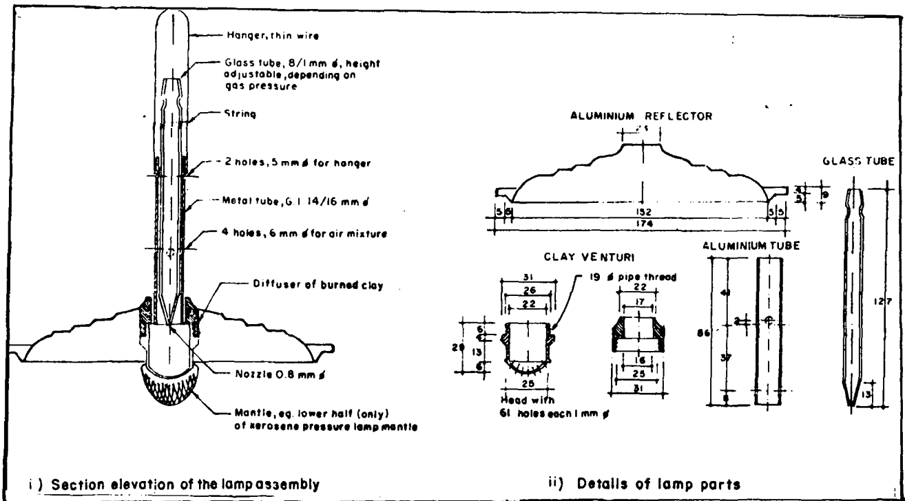
Fig. 57. Simple Biogas Lamp (China)
