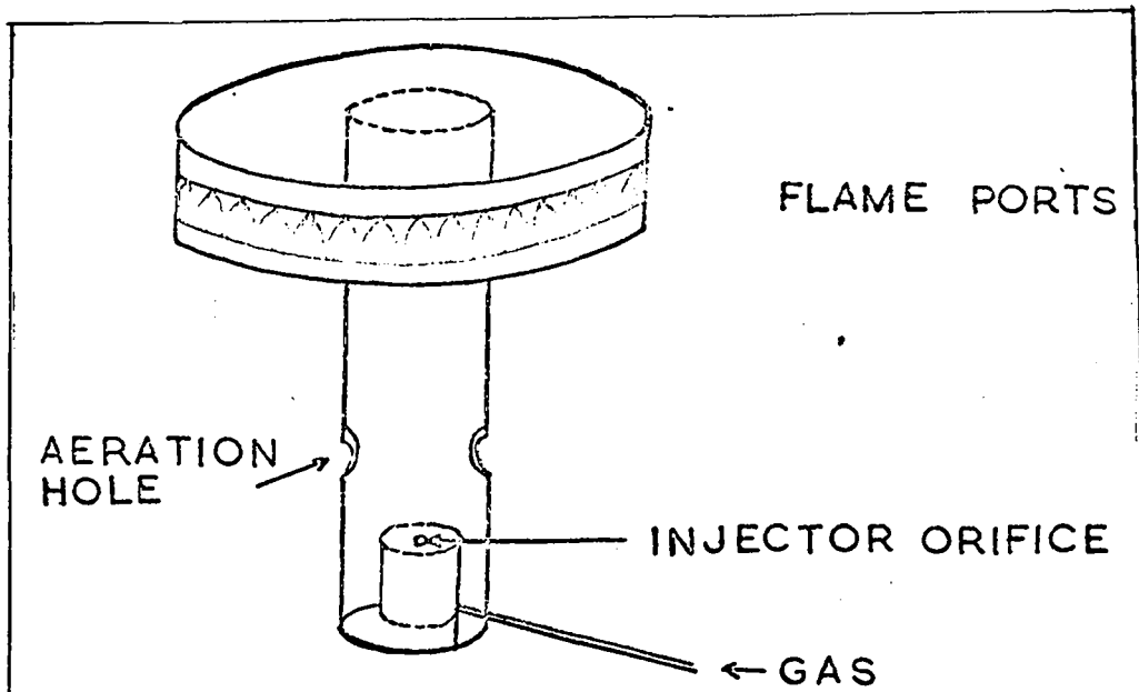
Fig. 37: Burner (Watson-type)
